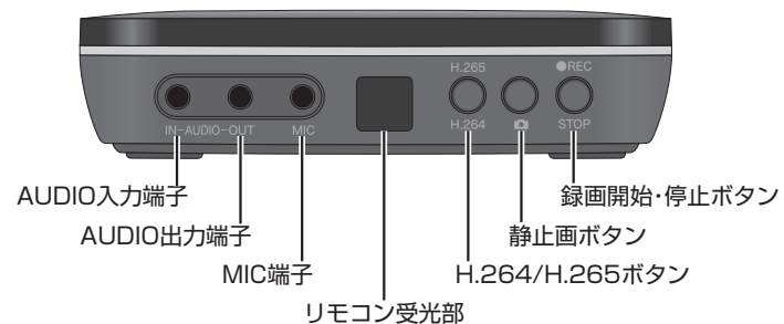
本体正面
